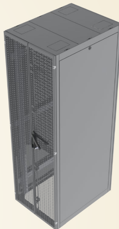
Gabinete Servidor 44U x L600 x P1000mm com porta frontal perfurada e porta traseira bipartida
