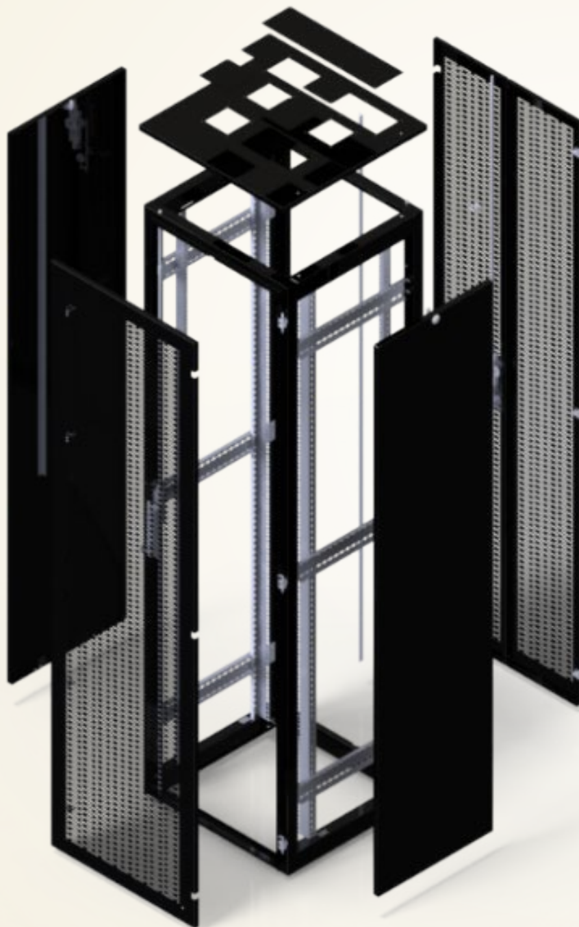
Visão explodida do rack
